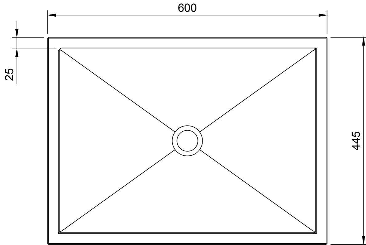
TOP
