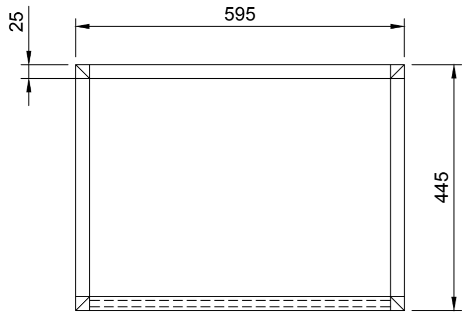
TOP
